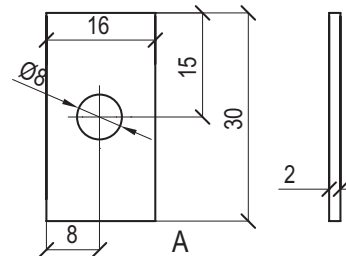
Шайба кронштейна крепежного
