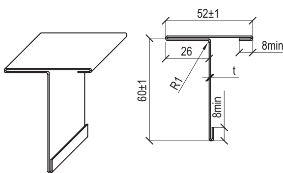
Крепежный профиль Т-образный 60x52x3000 КПТ-60x52x3000
