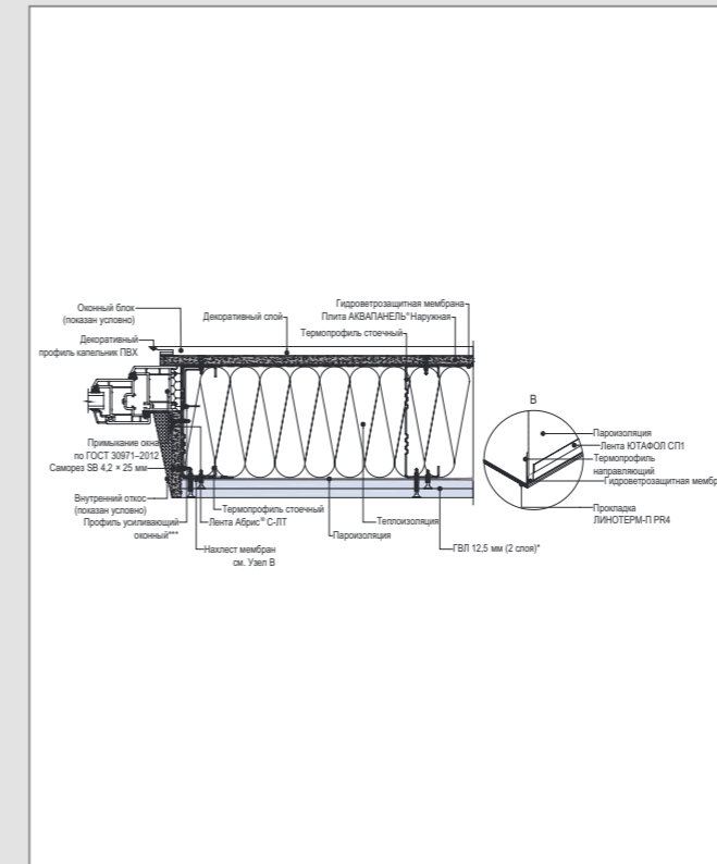
В 5 – Боковое примыкание к оконному блоку
