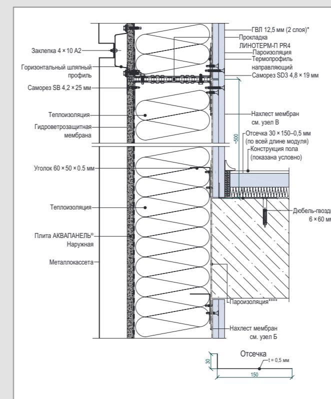
С 3 – Вертикальный разрез рядового модуля
