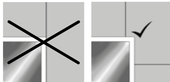
Рис. 22. Крепление плит в области проема
