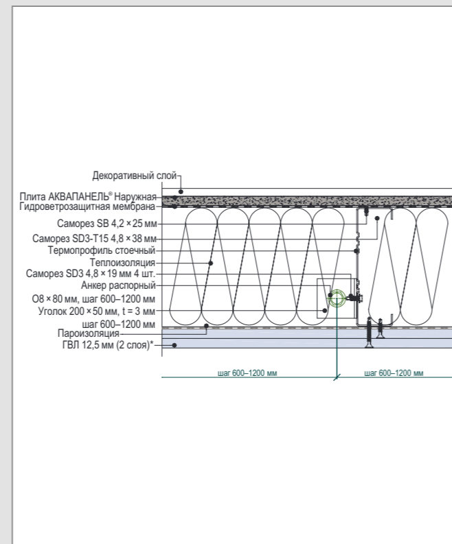
В 4 – Горизонтальный разрез рядового модуля. Примыкание к перекрытию. Вариант 2
