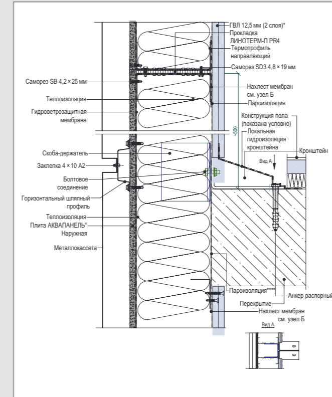
D 1 – Вертикальный разрез рядового модуля. Крепление к перекрытию
