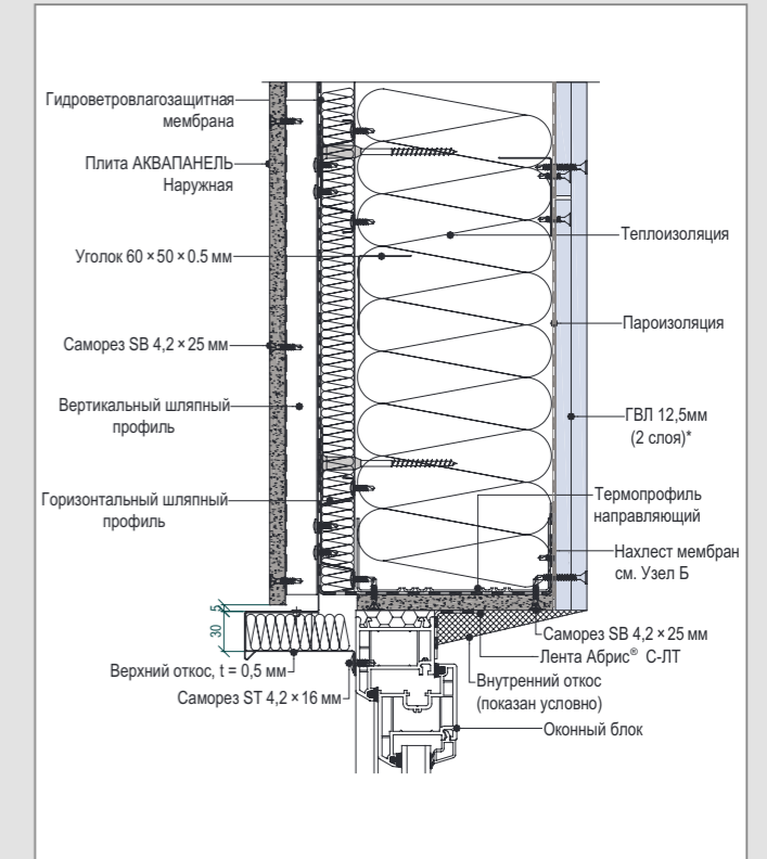
А 6 – Верхнее примыкание к оконному блоку
