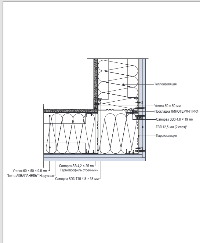
В 9 – Внутренний угол
