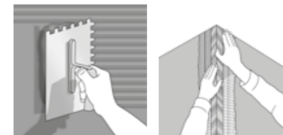
Рис. 27. Армирование углов
