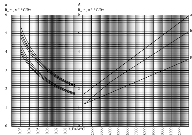
Рис. 14. Приведенное сопротивление теплопередаче стен ( R_{0}^{np} ) с каркасом из термопрофилей толщиной: 0,7 (1); 1,0 (2); 1,2 (3) и 1,5 (4) мм при толщине теплоизоляции 150 (I) и 200 (II) мм в зависимости от расчетного значения коэффициента теплопроводности теплоизоляции ( \lambda ) в сравнении с требуемыми ( R_{0}^{np} ) из условия энергосбережения значениями сопротивления теплопередаче наружных КОС с применением ЛСТК в зданиях: жилых (А), общественных (Б) и производственных (В), в зависимости от расчетных значений градусо-суток отопительного периода (ГСОП)
