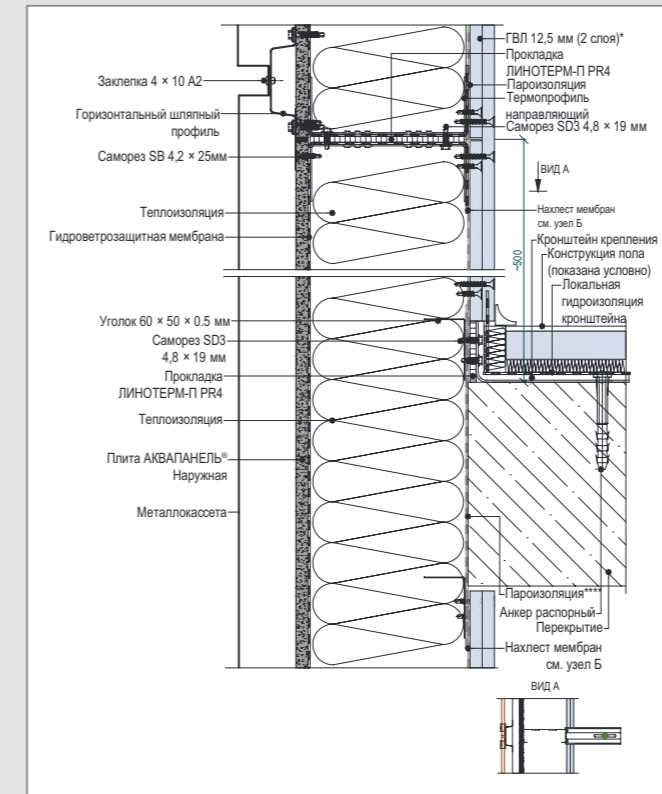
С 1 – Вертикальный разрез рядового модуля. Крепление к перекрытию
