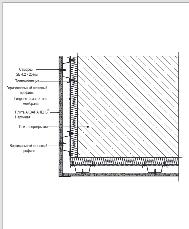
А 3 – Горизонтальный разрез внешнего угла по перекрытию
