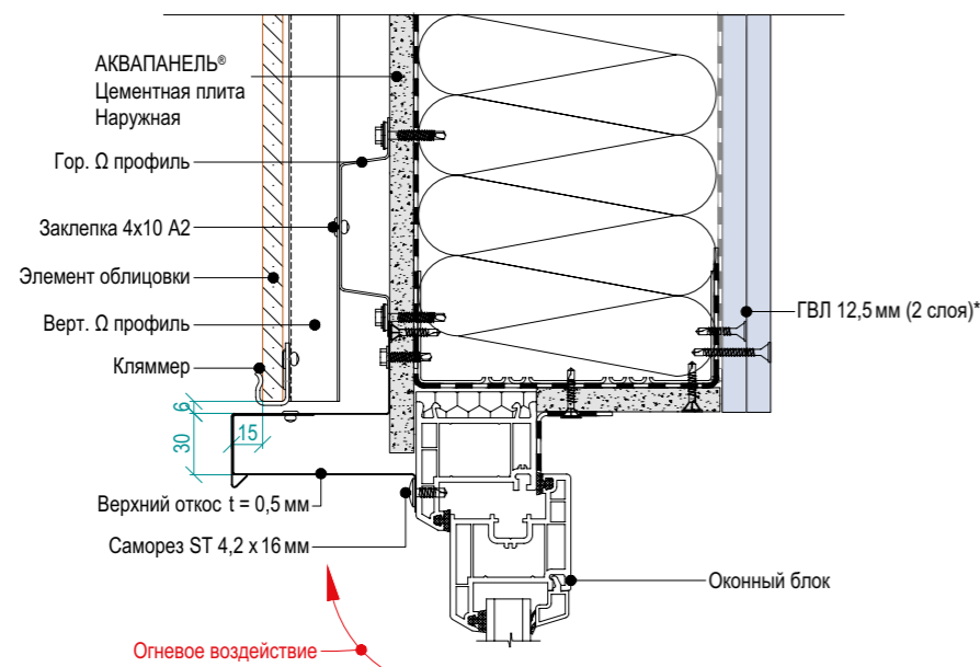
Рис. 8а. Пример узла верхнего откоса с противопожарной отсечкой пламени огня
