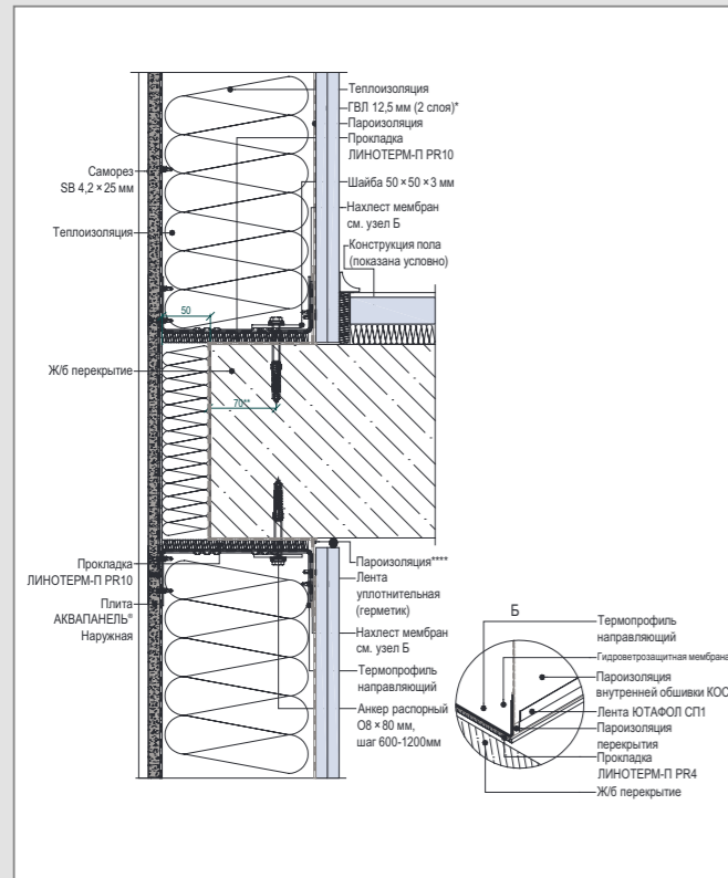
В 1 – Вертикальный разрез рядового модуля. Примыкание к перекрытию
