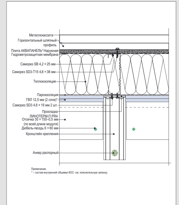
С 2 – Горизонтальный разрез рядового модуля. Крепление к перекрытию
