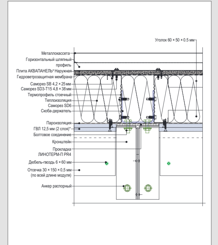
D 2 – Горизонтальный разрез рядового модуля. Крепление к перекрытию
