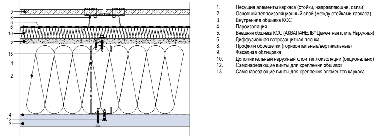
Рис. 2. Основные компоненты наружной каркасно-обшивной стены
