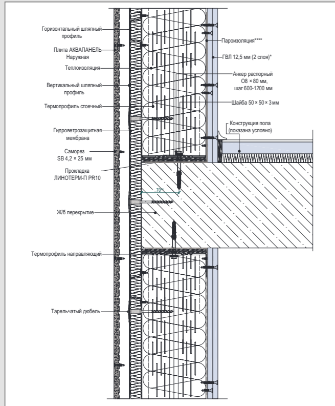
А 1 – Вертикальный разрез рядового модуля. Примыкание к перекрытию
