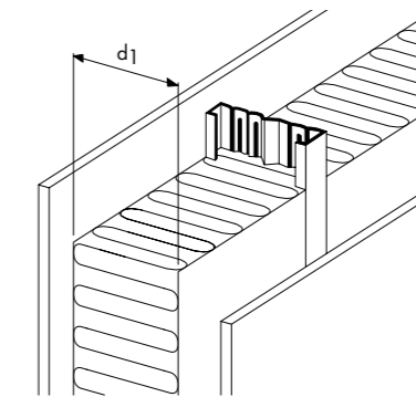
Рис. 13. Толщина утепляющего слоя наружной КОС с применением ЛСТК
