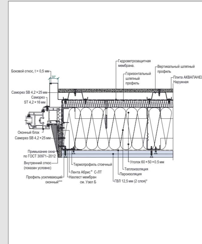
А 5 – Боковое примыкание к оконному блоку
