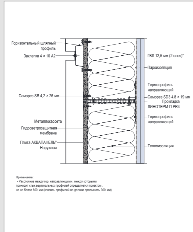
C 6 – Горизонтальный стык смежных модулей
