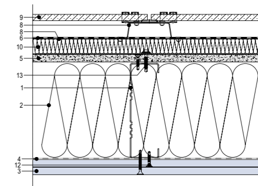
Рис. 8. Тип № 3. Схема конструктивного исполнения наружной несущей КОС с зазором и дополнительным наружным утеплением (расшифровку цифровых обозначений см. в табл. 1)
