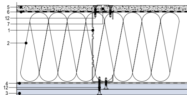
Рис. 6. Тип № 1. Схема конструктивного исполнения наружной несущей КОС без зазора с внешней стороны (расшифровку цифровых обозначений см. в табл. 1)
