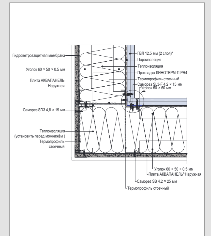
В 8 – Внешний угол
