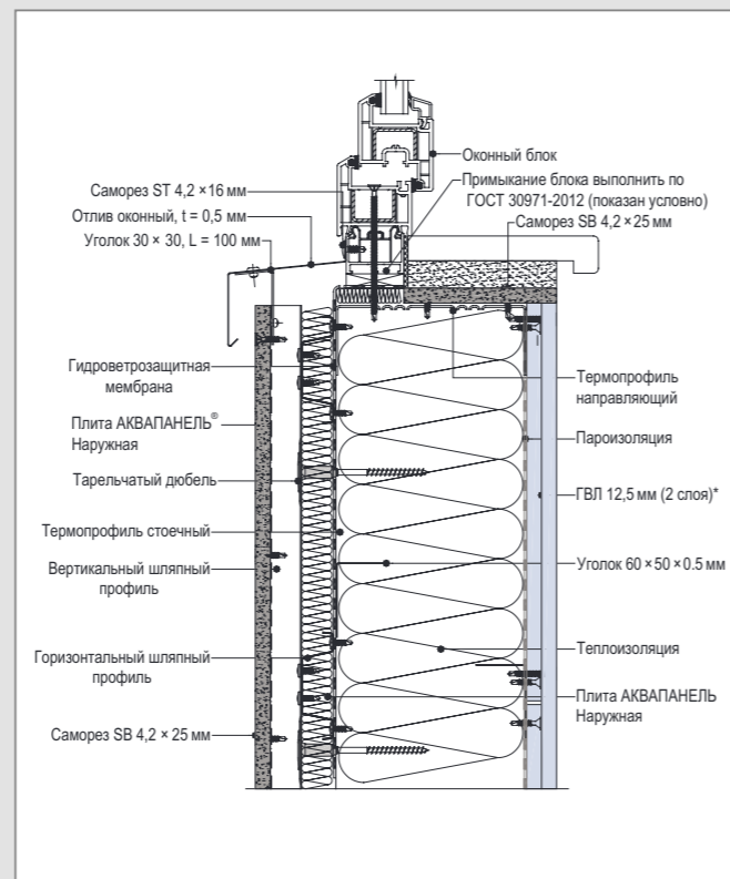
А 4 – Нижнее примыкание к оконному блоку
