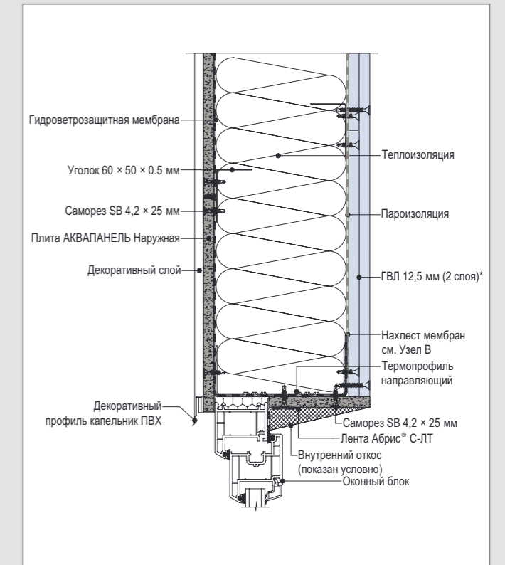
В 6 – Верхнее примыкание к оконному блоку
