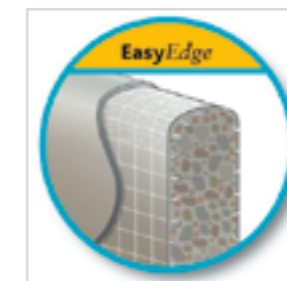
Рис. 15. Продольная кромка плит
