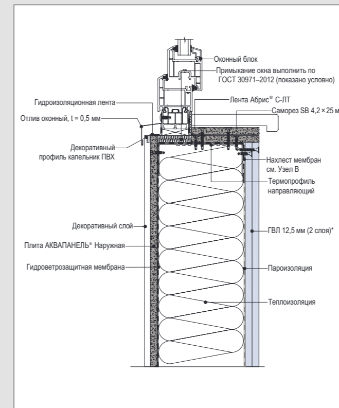
В 7 – Нижнее примыкание к оконному блоку
