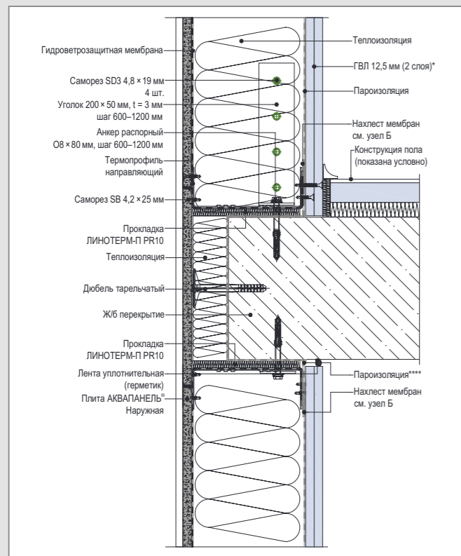
В 3 – Вертикальный разрез рядового модуля. Примыкание к перекрытию. Вариант 2.
