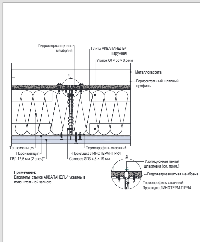
C 6 – Вертикальный стык смежных модулей
