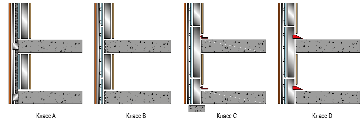
Рис. 5. Классификация наружных несущих стен в зависимости от типа примыкания к несущим конструкциям здания
