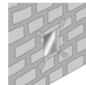
Рис. 28. Армирование облицовки в углах оконных и дверных проемов
