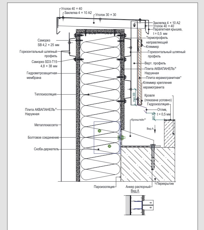
D 4 – Крепление к плите покрытия. Паранет
