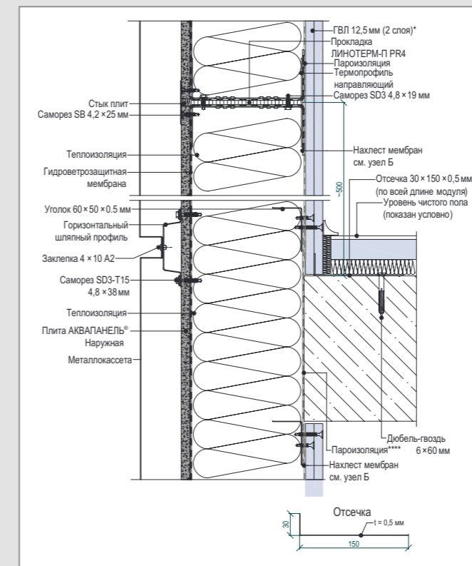
D 3 – Вертикальный разрез рядового модуля
