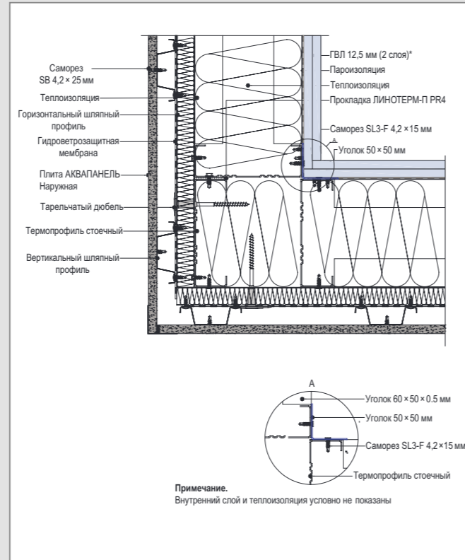
А 2 – Горизонтальный разрез внешнего угла
