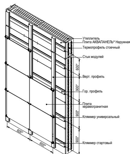
* размеры уточняются в рабочем проекте Рис. 1. Общий вид наружной каркасно-обшивной стены (КОС)
