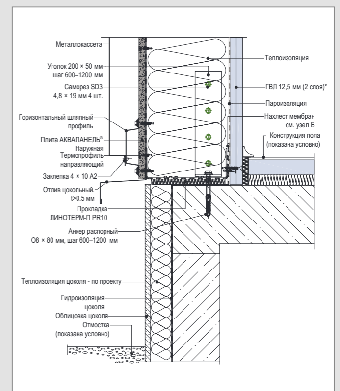
С 4 – Примыкание к фундаменту. Вариант 1
