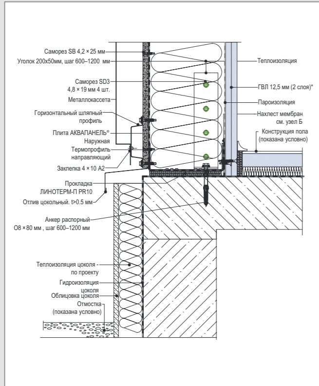
C 5 – Примыкание к фундаменту. Вариант 2
