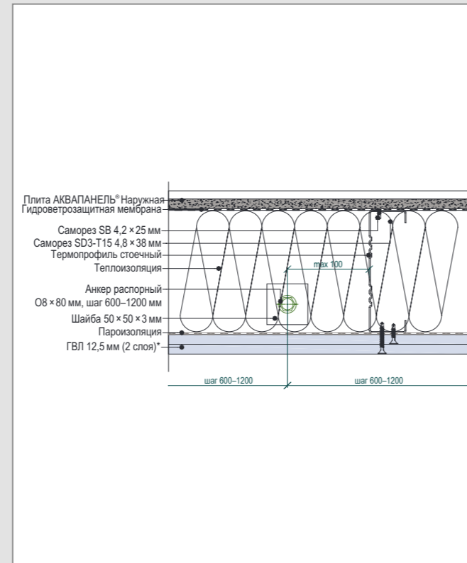
В 2 – Горизонтальный разрез рядового модуля. Примыкание к перекрытию.
