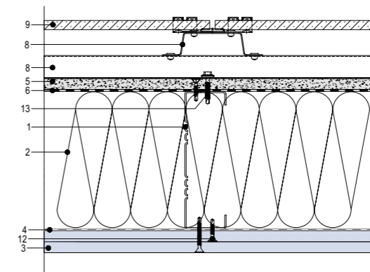
Рис. 7. Тип № 2. Схема конструктивного исполнения наружной несущей КОС с зазором с внешней стороны (расшифровку цифровых обозначений см. в табл. 1)
